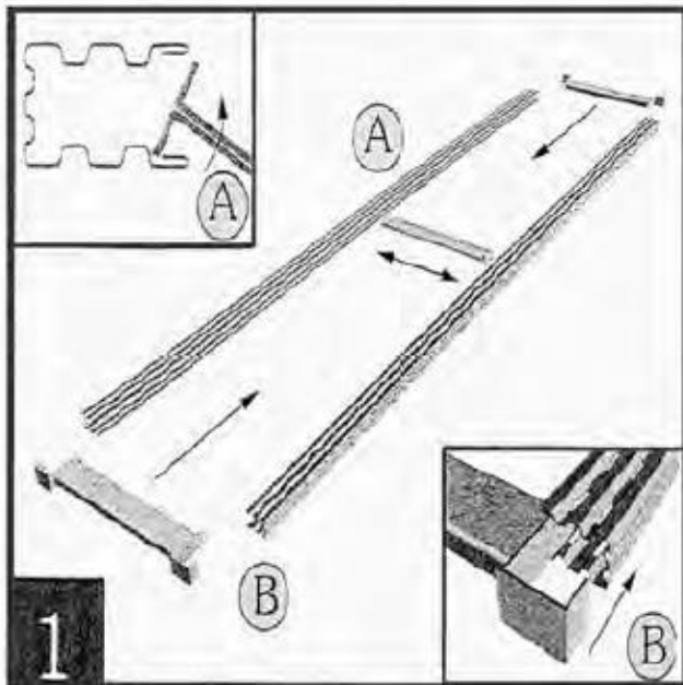
Рис.1 Сборка стоек (рамок)
