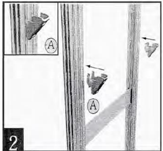
Рис.2 Установка кронштейнов для полок
